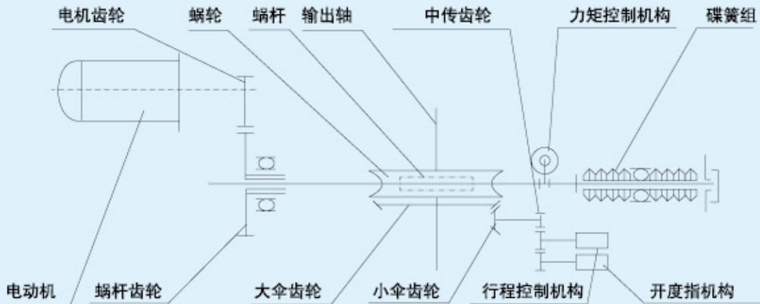
图4 传动原理图
