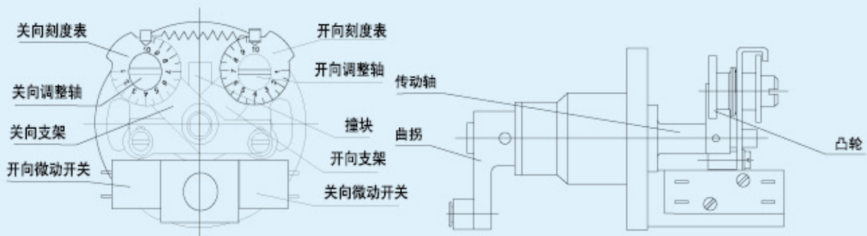
图5 力矩控制机构
